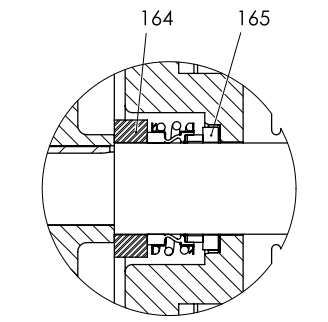
Mechanical Seal Application Mekanik Salmastra Uygulaması
