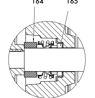
Mechanical Seal Application Mekanik Salmastra Uygulaması
